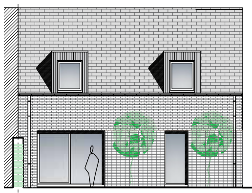
Zijgevel links
