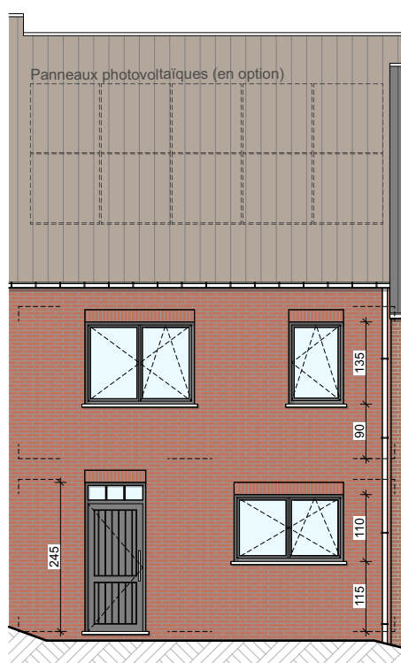
Façade avant
