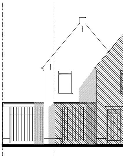
Voorgevel
