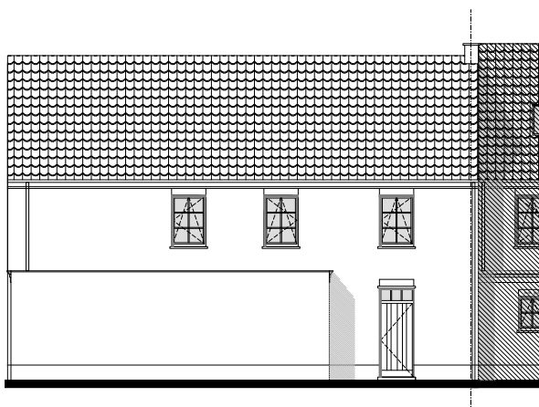
Zijgevel links
