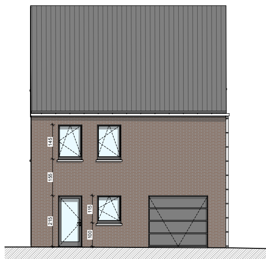
Façade avant
