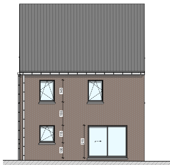
Façade arrière
