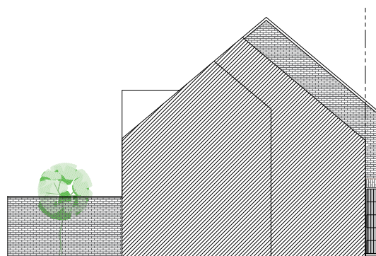
Vorgevel
