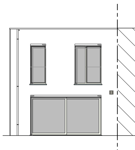
Achtergevel
