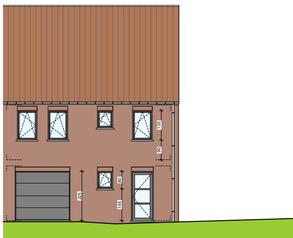
Façade avant
