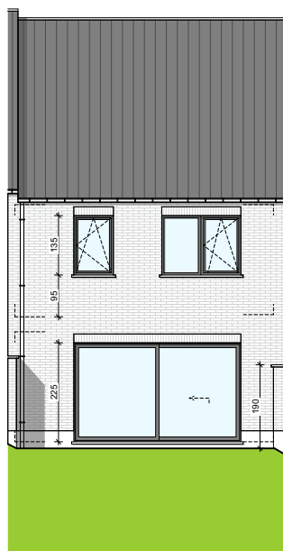
Façade arrière
