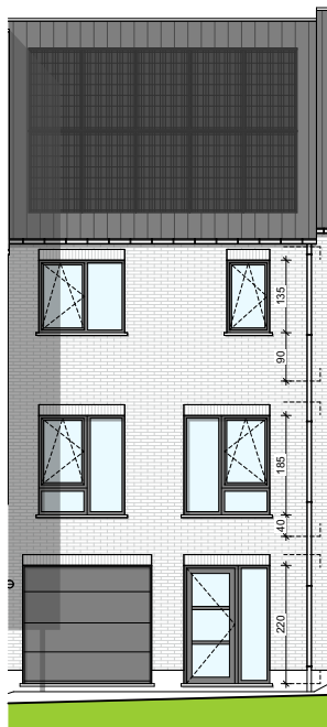
Façade avant
