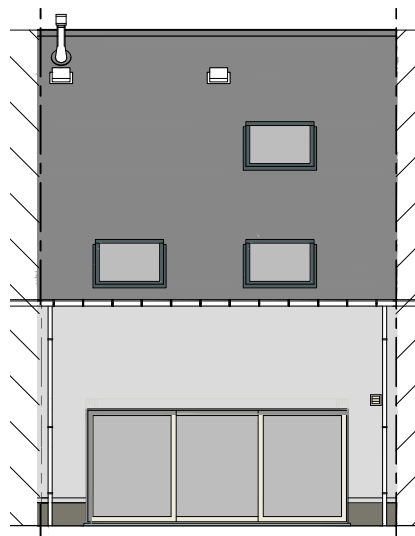
Achtergevel
