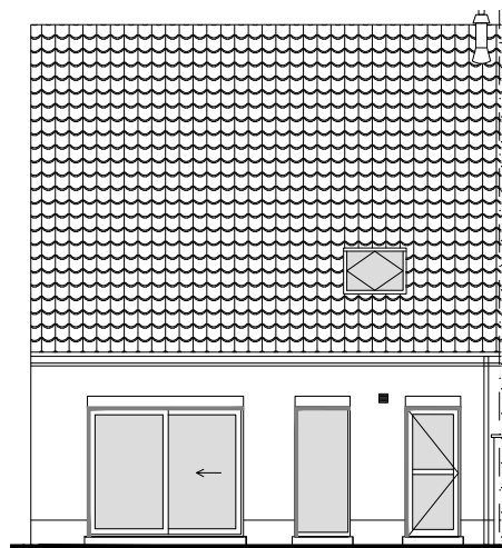
Achtergevel
