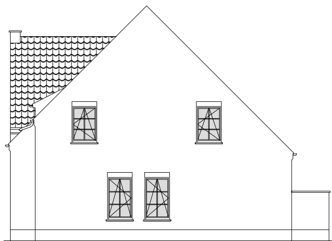
Zijgevel rechts
