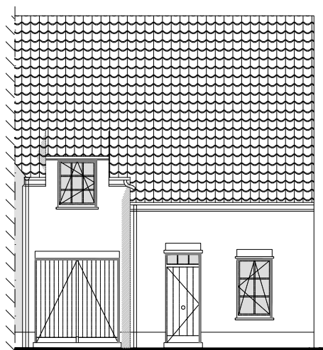
Voorgevel
