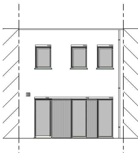
Vorgevel
