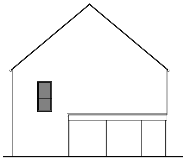
Zijgevel rechts
