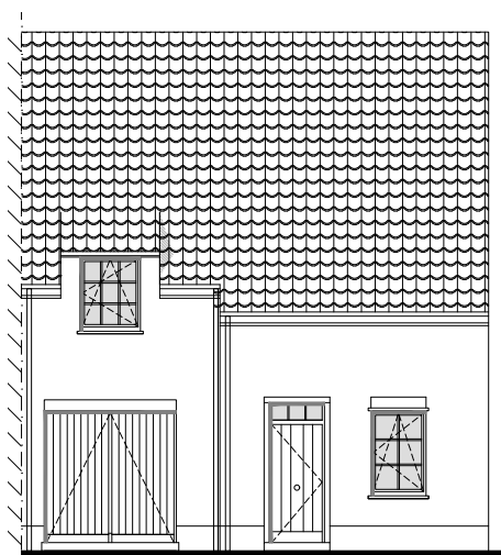
Voorgevel
