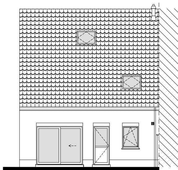
Achtergevel
