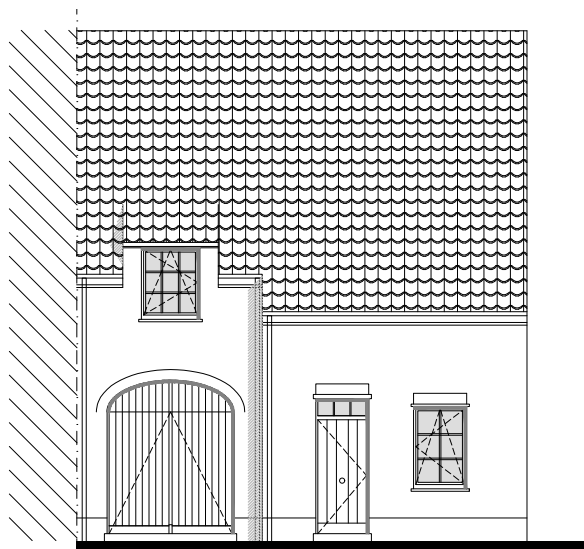
Voorgevel
