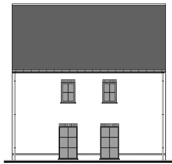
Zijgevel rechts
