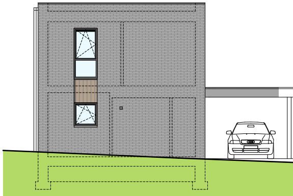
Façade avant
