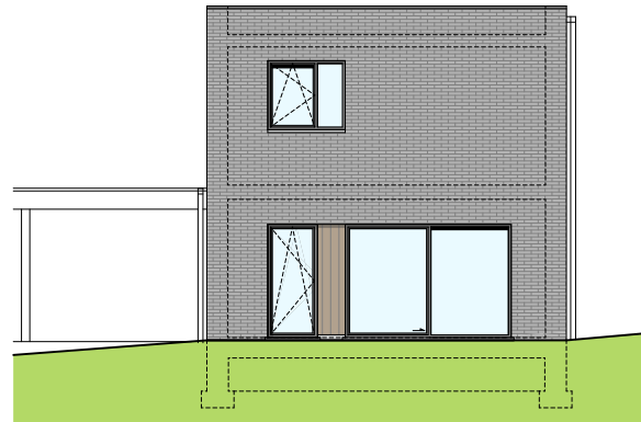
Façade arrière
