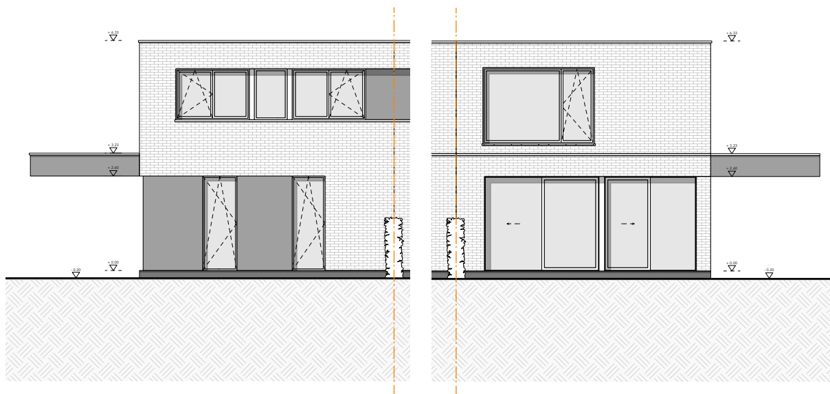
Voorgevel
