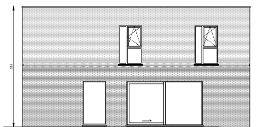
Zijgevel links
