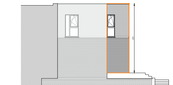
Zijgevel rechts
