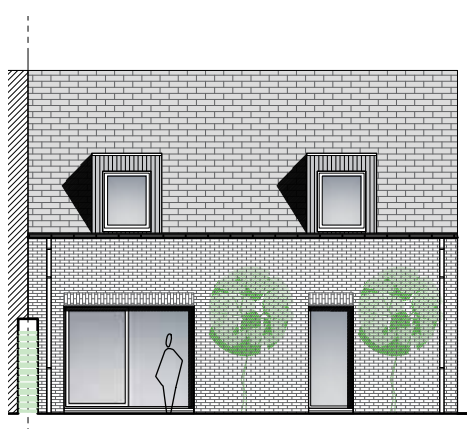
Zijgevel links
