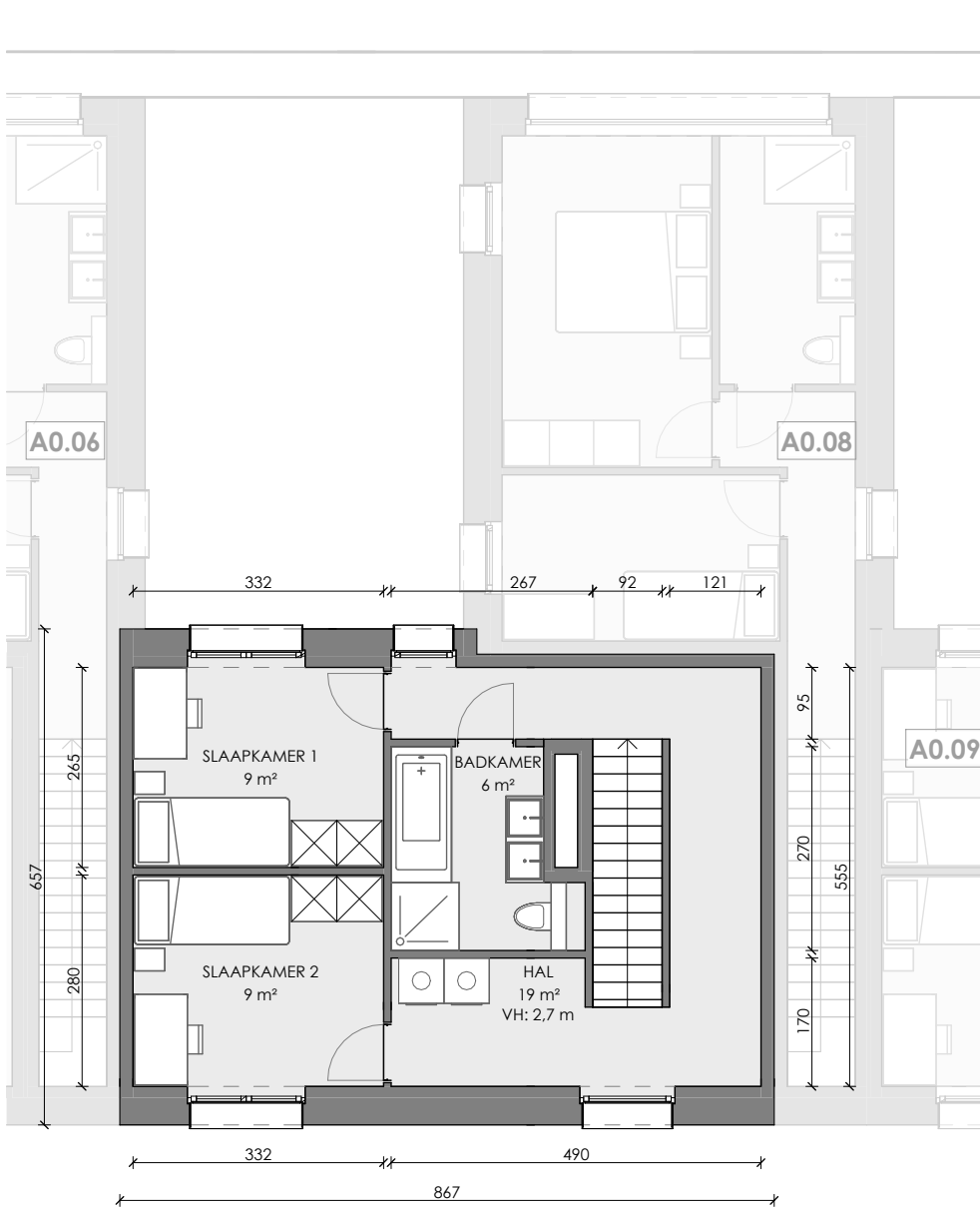
EERSTE VERDIEPING
