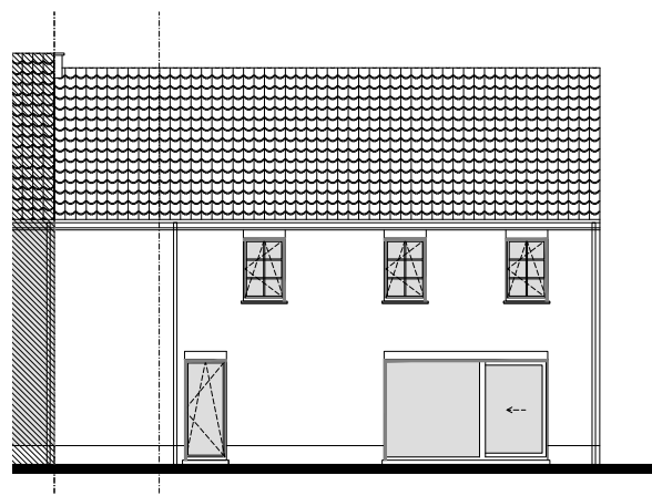
Zijgevel rechts
