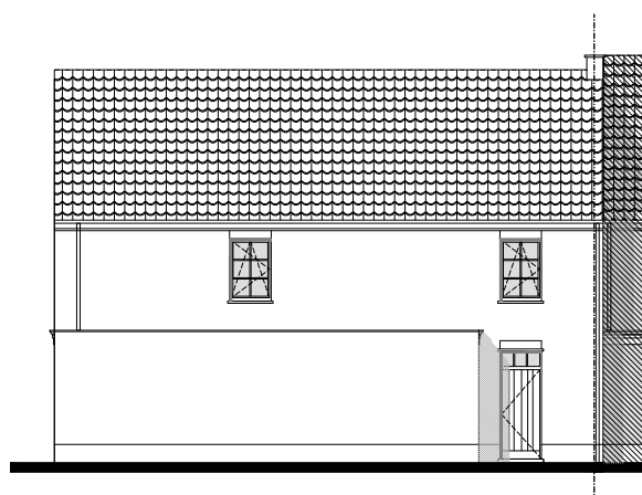
Zijgevel links
