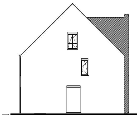
Zijgevel links
