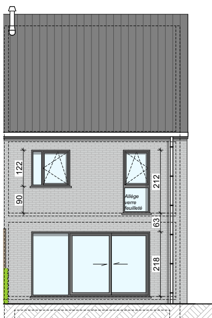
Façade arrière
