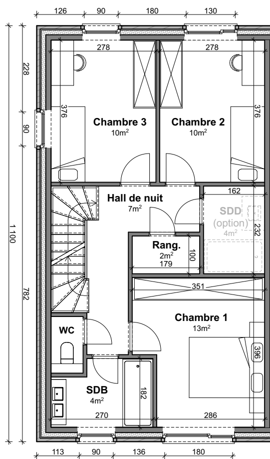
Etage
