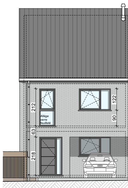
Façade avant
