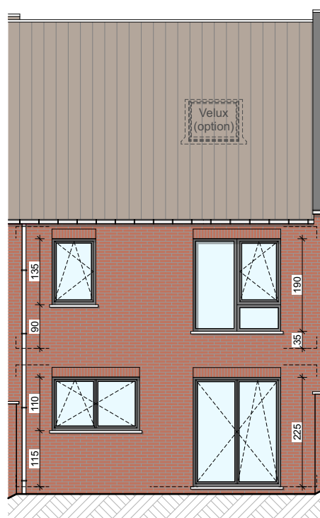
Façade arrière
